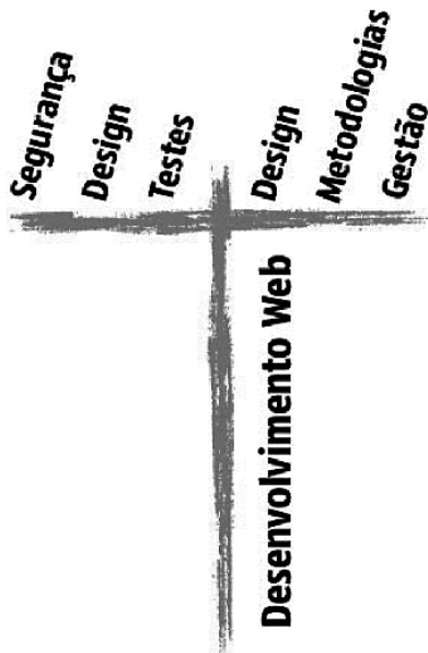
Figura 6.4: Profissional T
