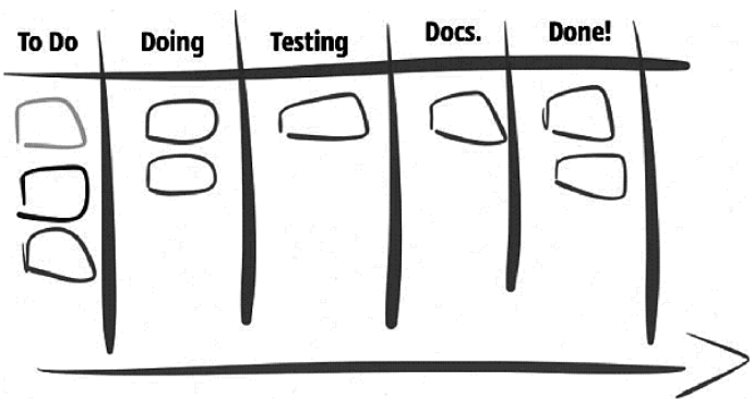
Figura 1.4: Kanban
