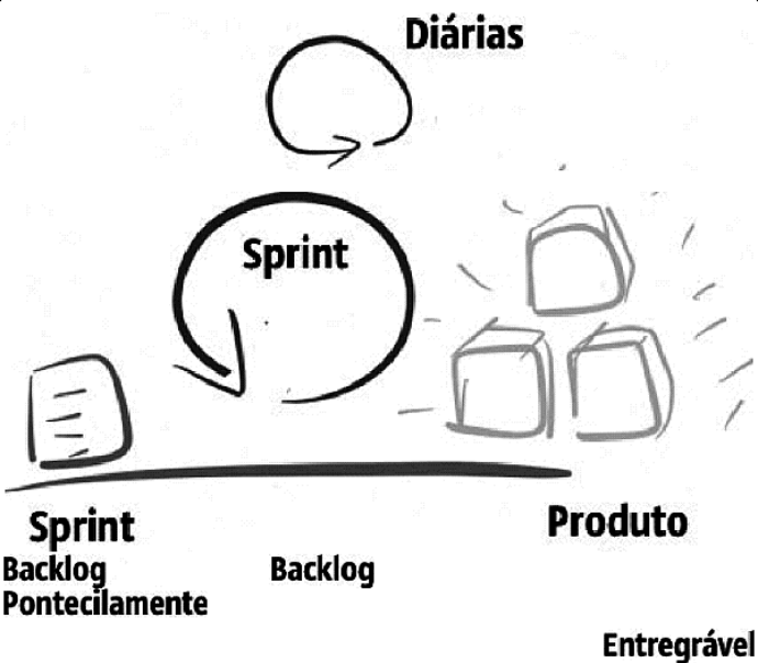
Figura 1.3: Scrum
